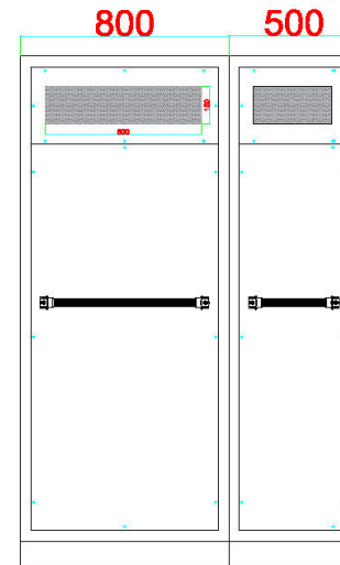
PANO ARKA GÖRÜNÜŞÜ
