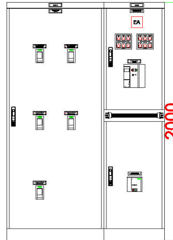
PANO ÖN GÖRÜNÜŞ
