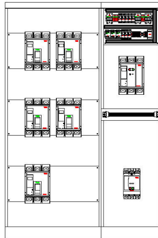
PANO İÇ GÖRÜNÜŞÜ
